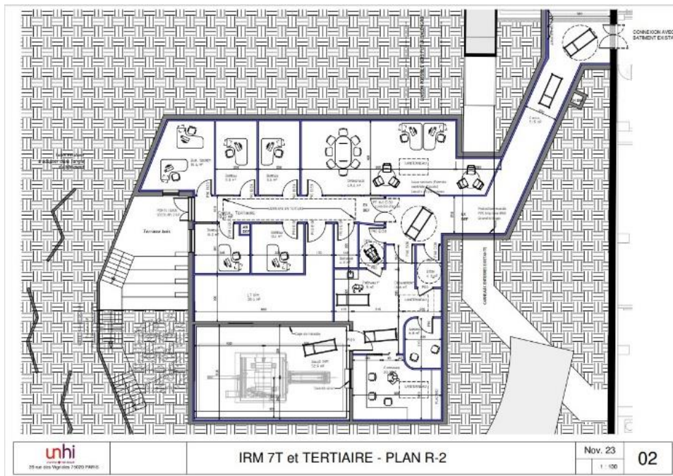
Plans de la future d'implantation de l'IRM 7T, à l'ouest de l'entrée de l'Hôpital Roger Salengro
